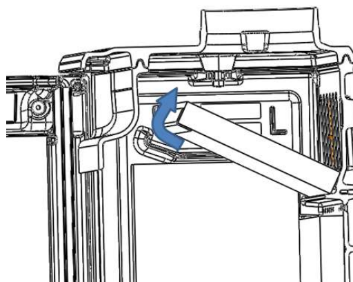
Figure No.11 - Otáčení výztuže
