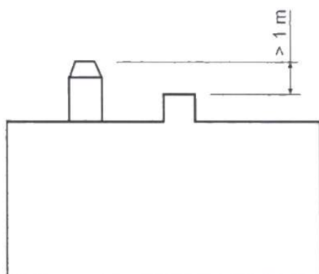
Figure No.5 - Vzdálenosti mezi korunou komína a hřebenem střechy
