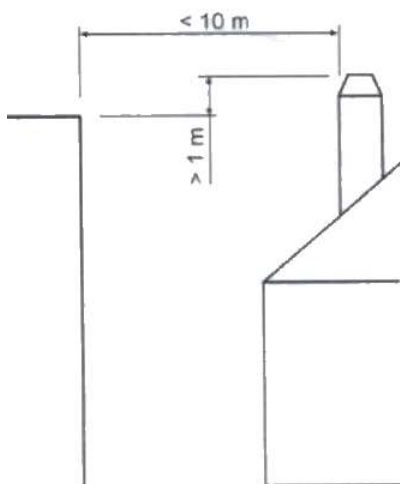
Figure No.6 - Vzdálenosti mezi korunou komína a objekty v okruhu 10 m
