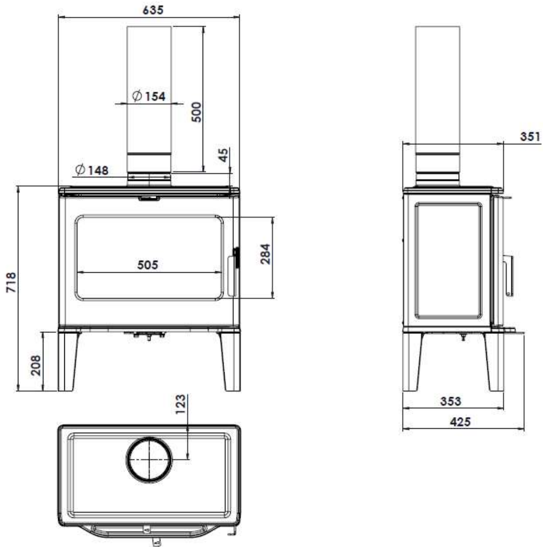
Figure No.1 - Rozměry spotřebiče Bidart v mm
