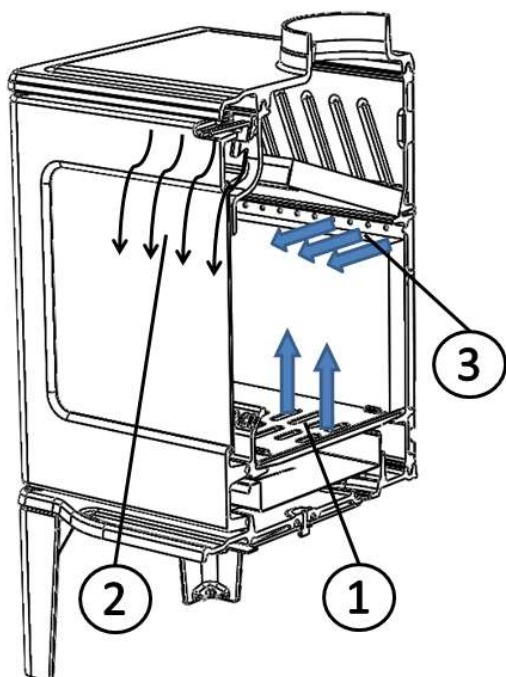
Figure No.10 - Přívody spalovacího vzduchu
