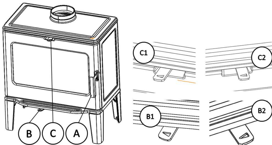
Figure No.9 - Provozní součásti spotřebiče
