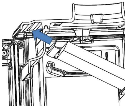
Figure No.12 - Uvolnění výztuže
