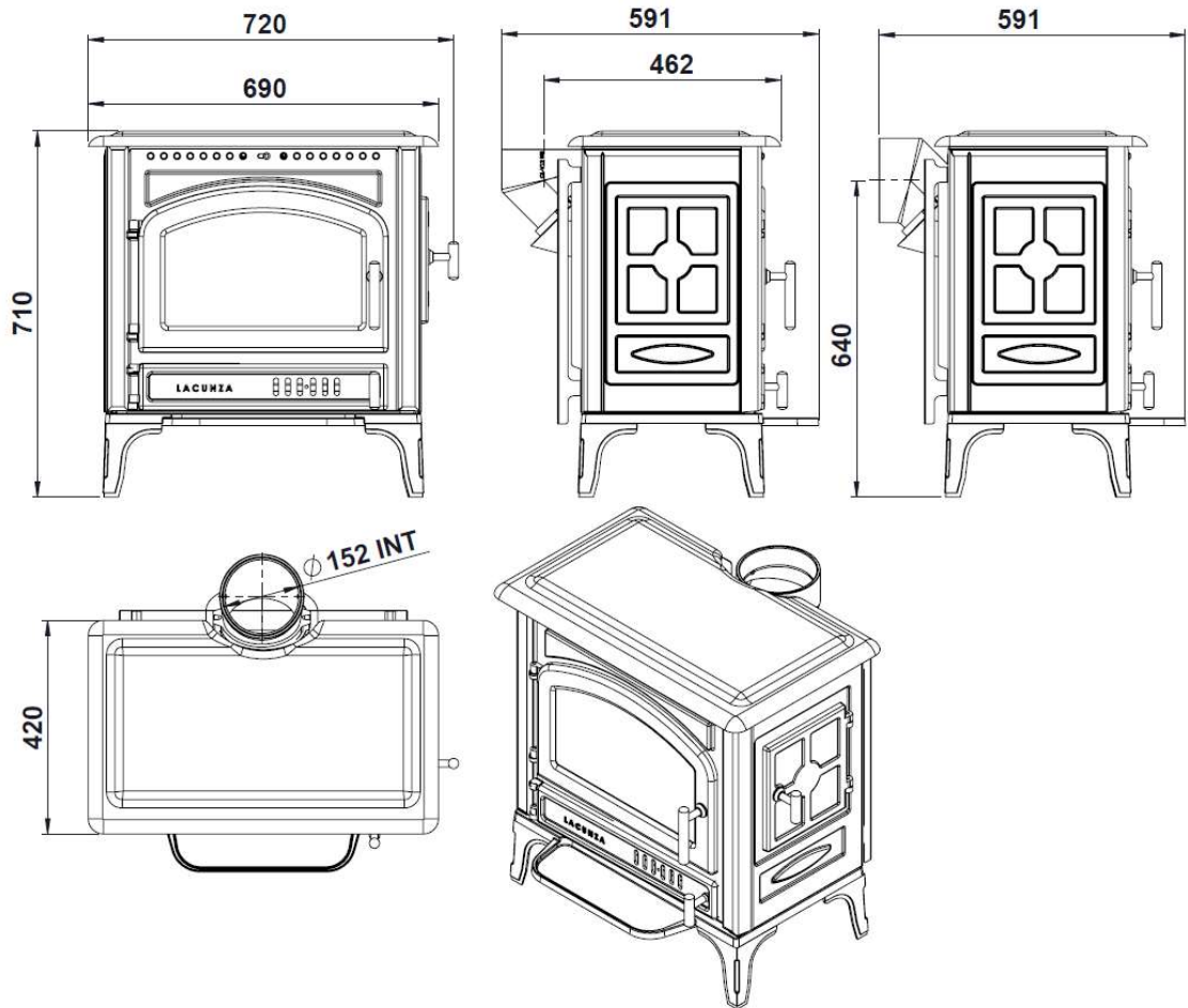
Figure No.1 - Rozměry spotřebiče Levante v mm
