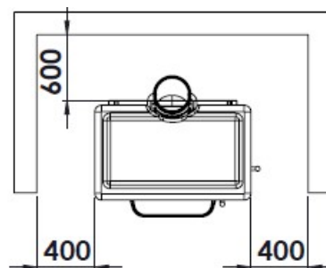
Figure No.3 - Bezpečnostní vzdálenosti
