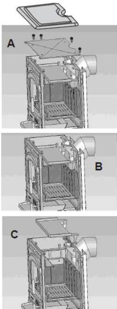
Figure No.10 - Demontáž deflektoru
