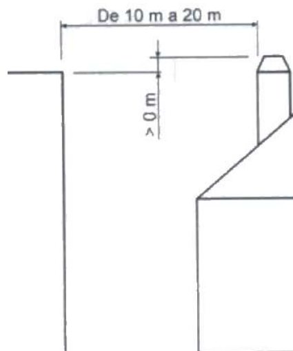
Figure No.4 - Vzdálenosti mezi korunou komína a objekty v okruhu 10 až 20 m.
