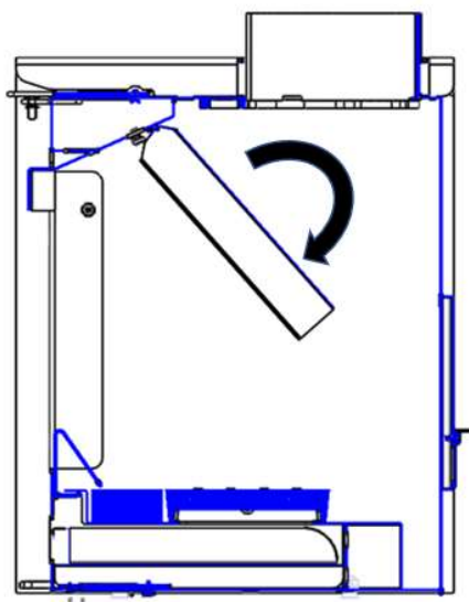
Figure No.13 - Otočení a sejmutí horního ocelového deflektoru
