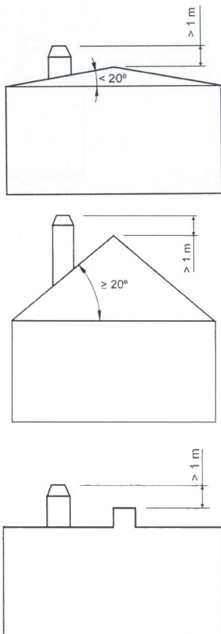
Figure No.2 - Vzdálenosti mezi korunou komína a hřebenem střechy
