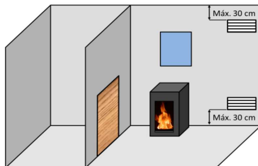
Figure No.1 - Směrné údaje pro větrací mřížky
