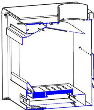
Figure No.12 - Vyjmutí zbytku vermikulitů z topeniště
