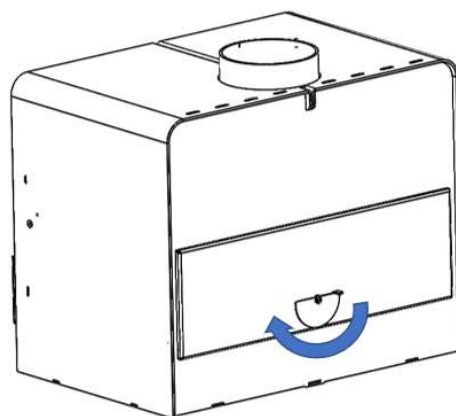
Figure No.9 - Uzavřené dvojitě sání spalovacího vzduchu
