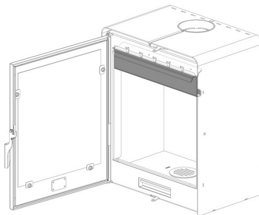
Figure No.5 - Příslušenství, které pomáhá v případě poklesu tlaku v důsledku špatného odvodu spalin
