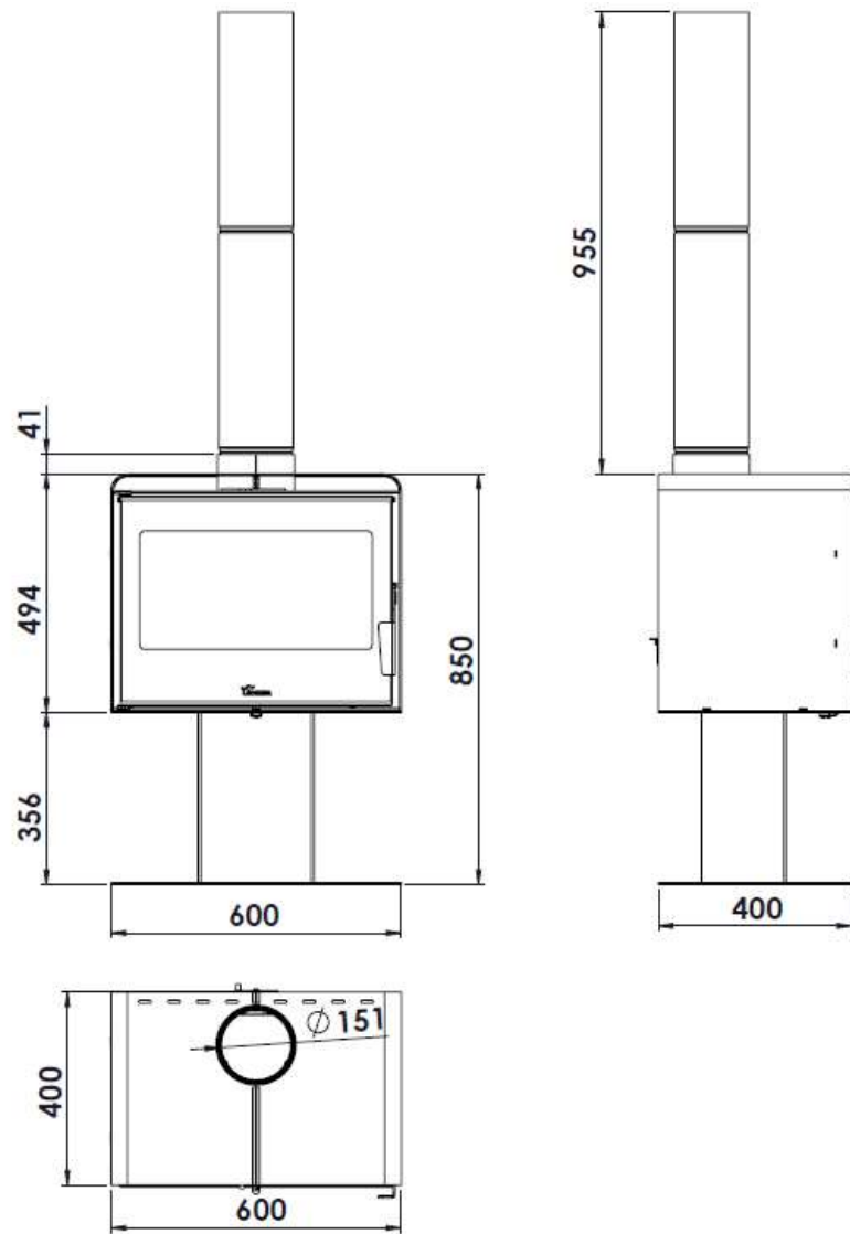
Figure No.1 - Rozměry řady Ocean/Atlantic v mm
